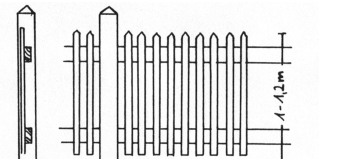
Staketzaun mit überragendem Pfosten
