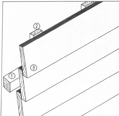
Horizontale Stulpschalung
