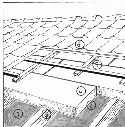
Abb. 72: Dachisolierung 1 Innere Dachbekleidung 2 Dampfbremse 3 Dachsparren 4 Wärmedämmung 5 wasserableitendes Unterdach 6 Dacheindeckung mit Unterkonstruktion
