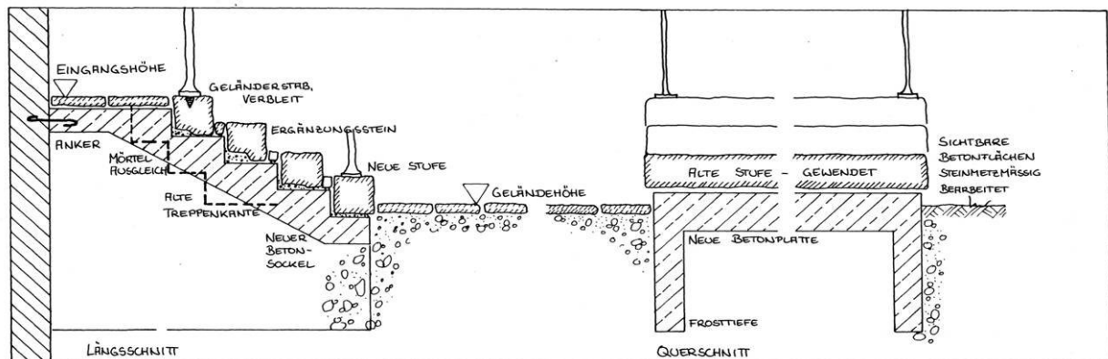
Abb. 83: Erneuerung einer Steintreppe
